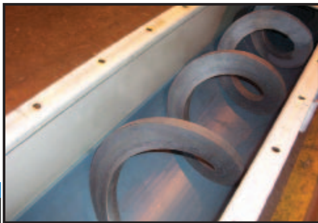
右：无轴螺旋会是解决众多问题的方案。
